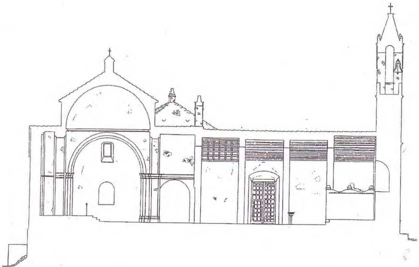
SECCION LONGITUDINAL 1
