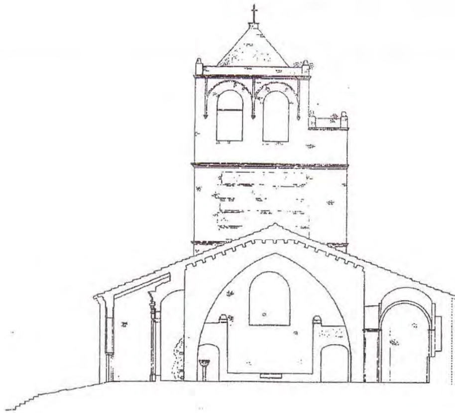
SECCIÓN TRANSVERSAL 2
