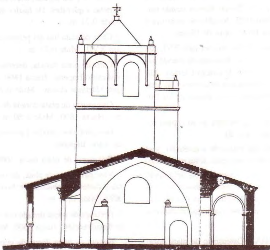
Sección c-d
