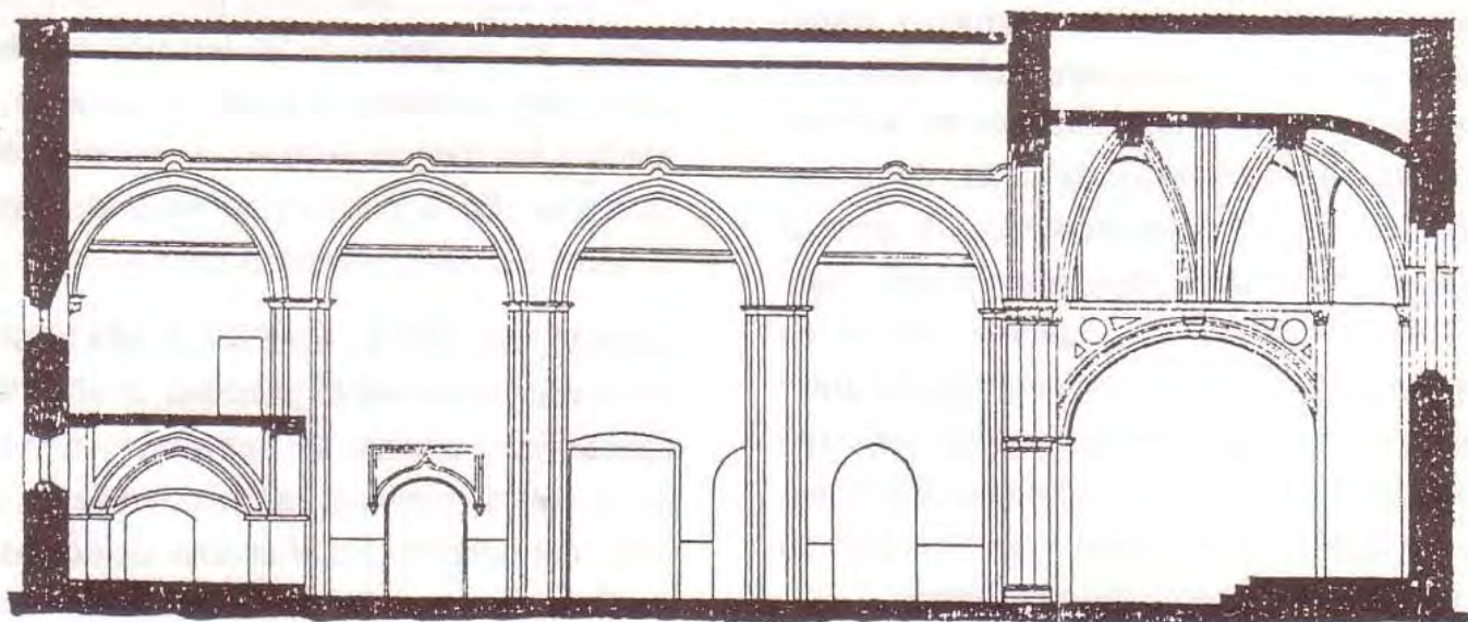
Sección a-b.
