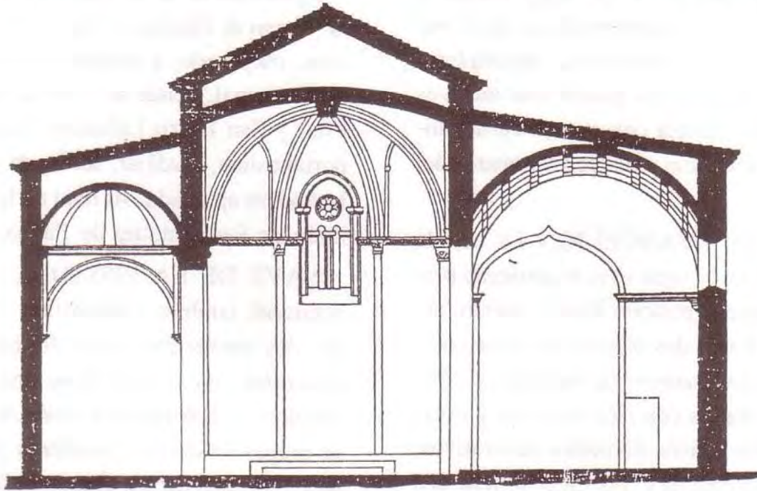
Sección c-d.
