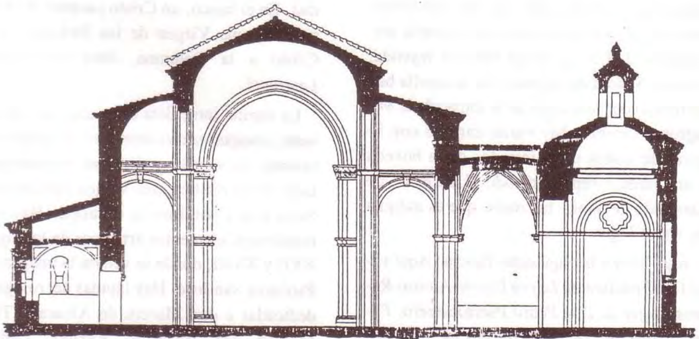
Sección e-f.
