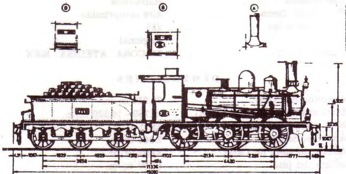
Locomotora serie 030 una de las que mas frecuentaron la Estación de GUADALCANAL. (Material Motor de la RENFE edición 1947)
